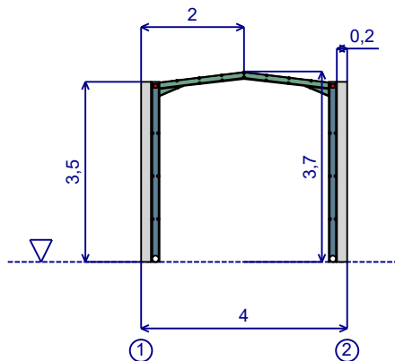
Figure 4 : Plan du portique B
