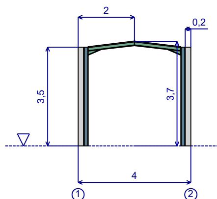
Figure 2 : Plan du portique représentatif
